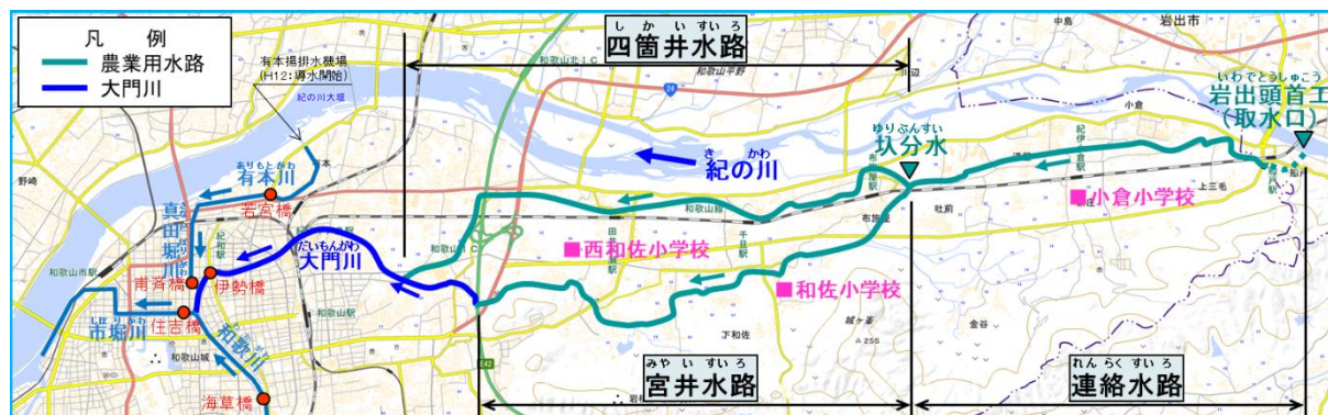
導水ルート図
